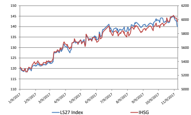
LS27 Index
